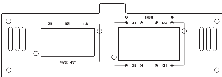
Схема №5 Схема подключения в «классическом» режиме, на нагрузку из 4-х динамиков.
