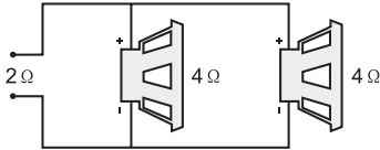
Параллельное соединение динамиков
