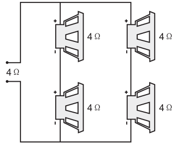
Последовательно-параллельное соединение динамиков
