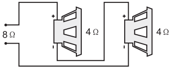
Последовательное соединение динамиков
